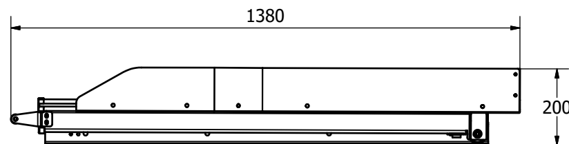
ภาพด้านข้าง SIDE VIEW
