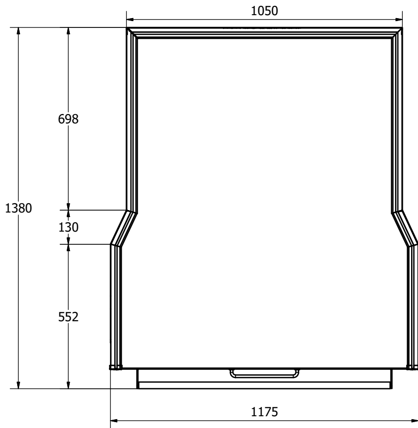
ภาพด้านบน TOP VIEW
